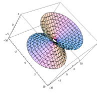
Hiper. Reglado ax^2 + by^2 - cz^2 - 1 = 0
