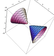
Hip. no Regl. ax^2 - by^2 - cz^2 - 1 = 0
