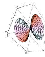
Cono ax^2 + by^2 - z^2 = 0
