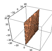
Plano doble x^2 = 0
